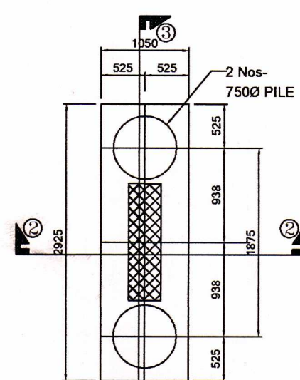
PILE - P2
