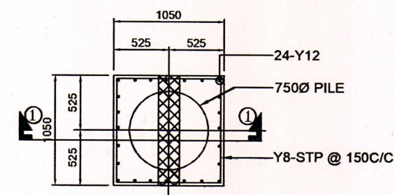
PILE-P1
