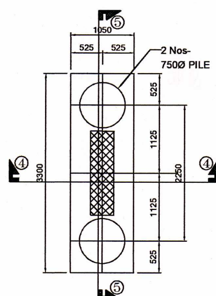
PILE - P2A
