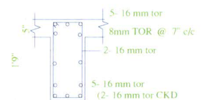
BEAM B5
