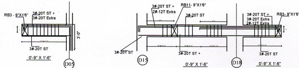
LONGITUDINAL SECTION OF GRID - D05
