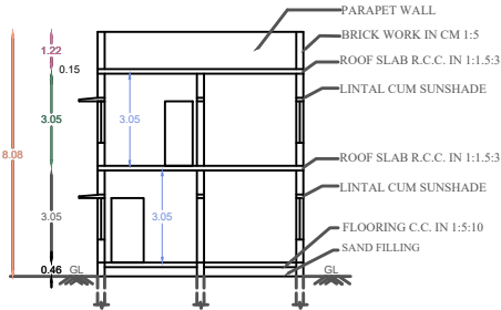
SECTION NO A-A
