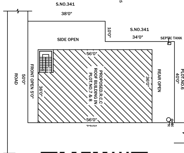
SITE PLAN SCALE: 1" = 16'0"
