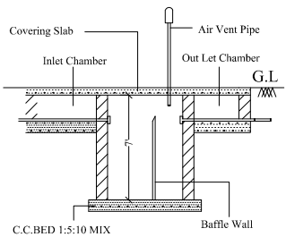
SECTION ON S.Tank [N.T.S.]
