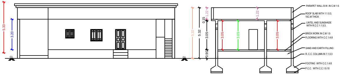
ELEVATION
