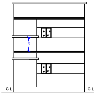
ELEVATION - A
