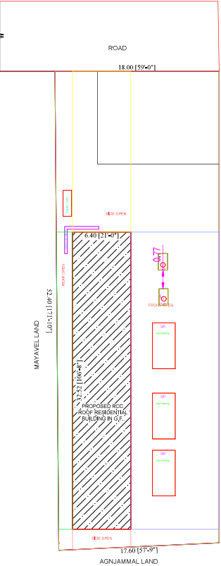
SITE PLAN 1:100
