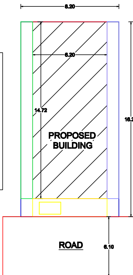
SITE PLAN 1:100 SCALE
