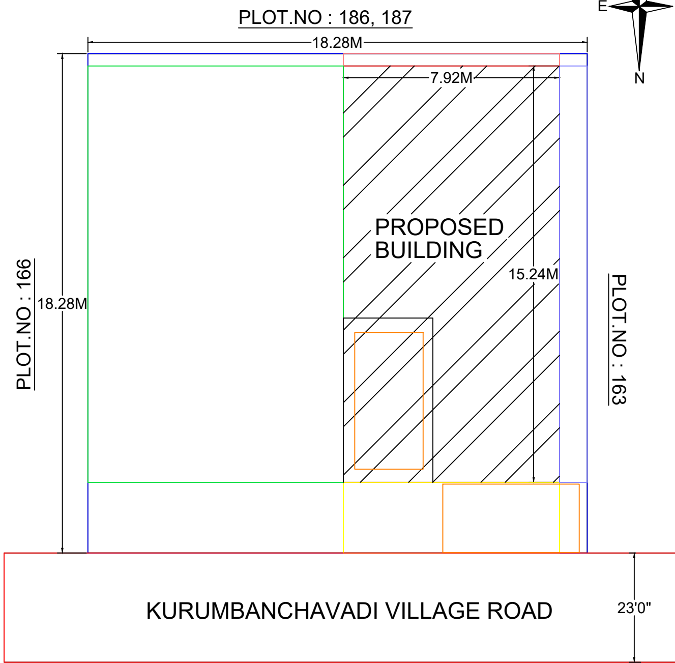
SITE PLAN 1:100 SCALE
