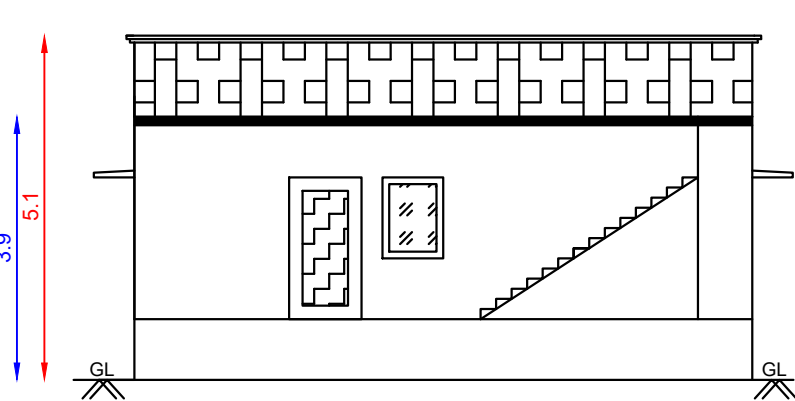
ELEVATION
