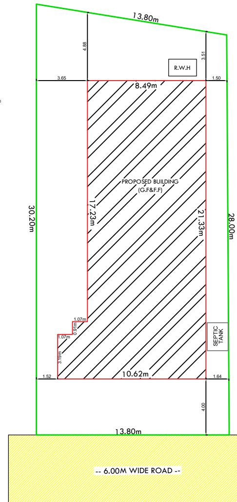
SITE PLAN (SCALE 1 : 100)
