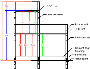
SECTION - AB
