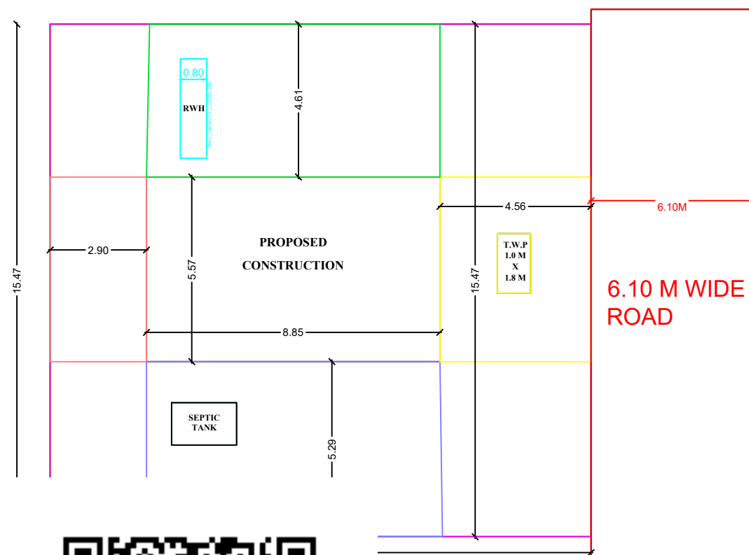
SITE PLAN SCALE : 1"= 8' OR [1 : 100]
