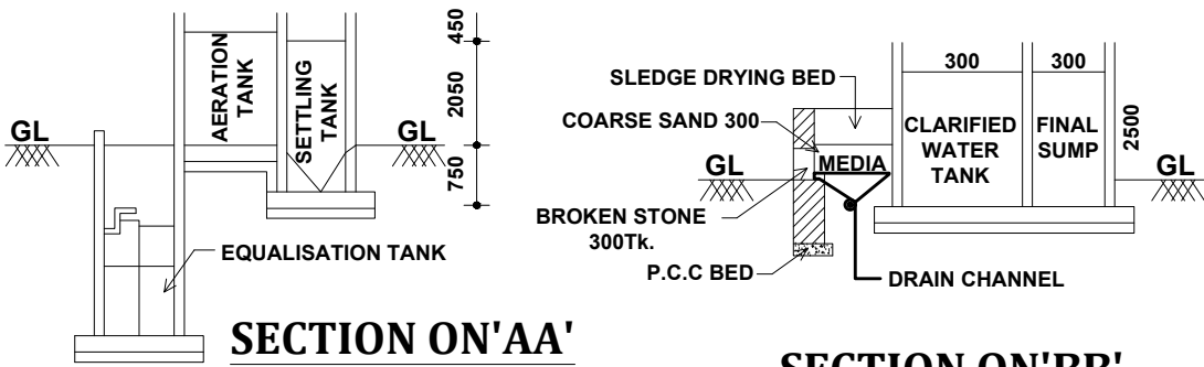
SECTION ON'BB'
