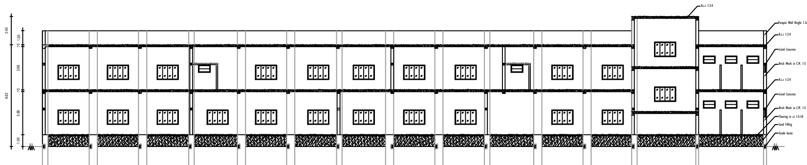
SECTION A-A
