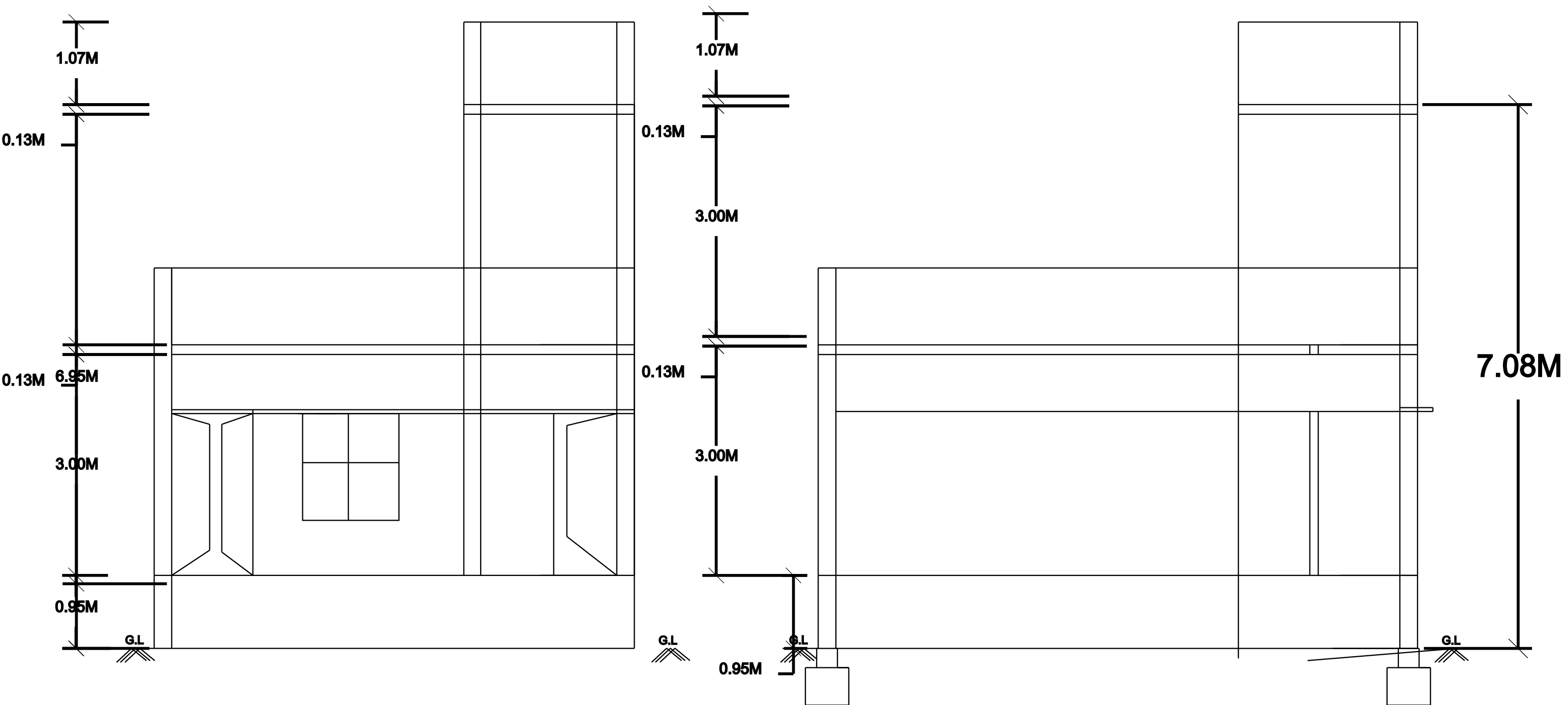
ELEVATION
