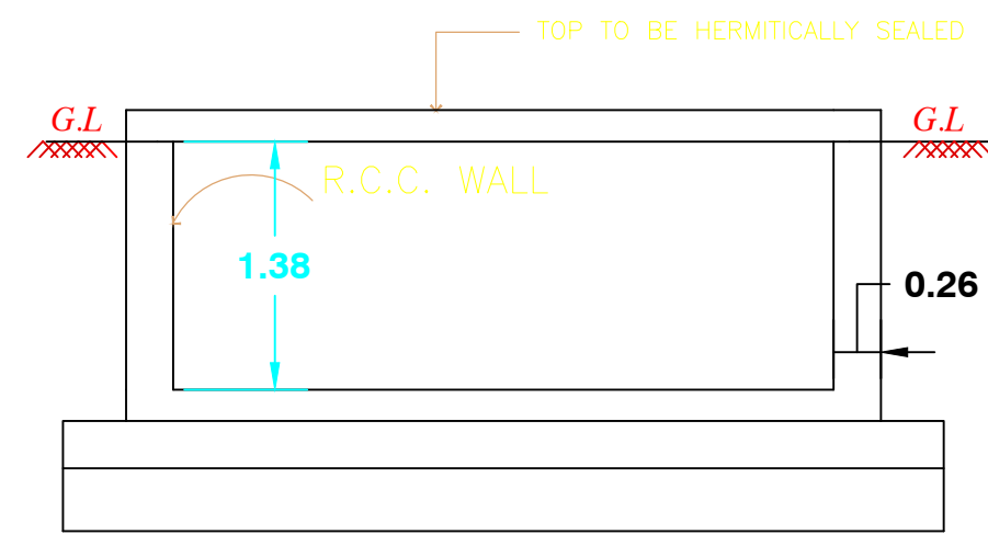
RWK SECTION (SAMPLE)
