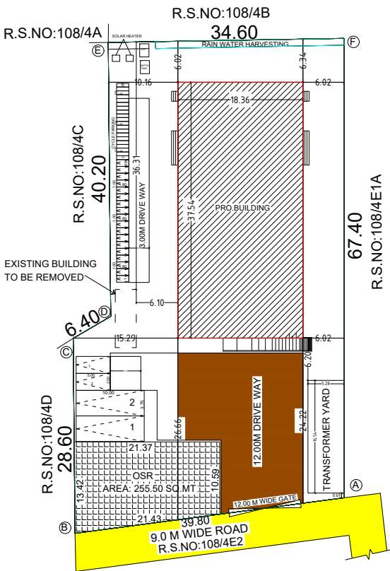
SITEPLAN SCALE:1:200
