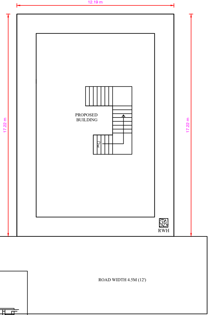
SITE PALN
