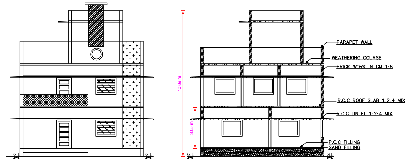
ELEVATION
