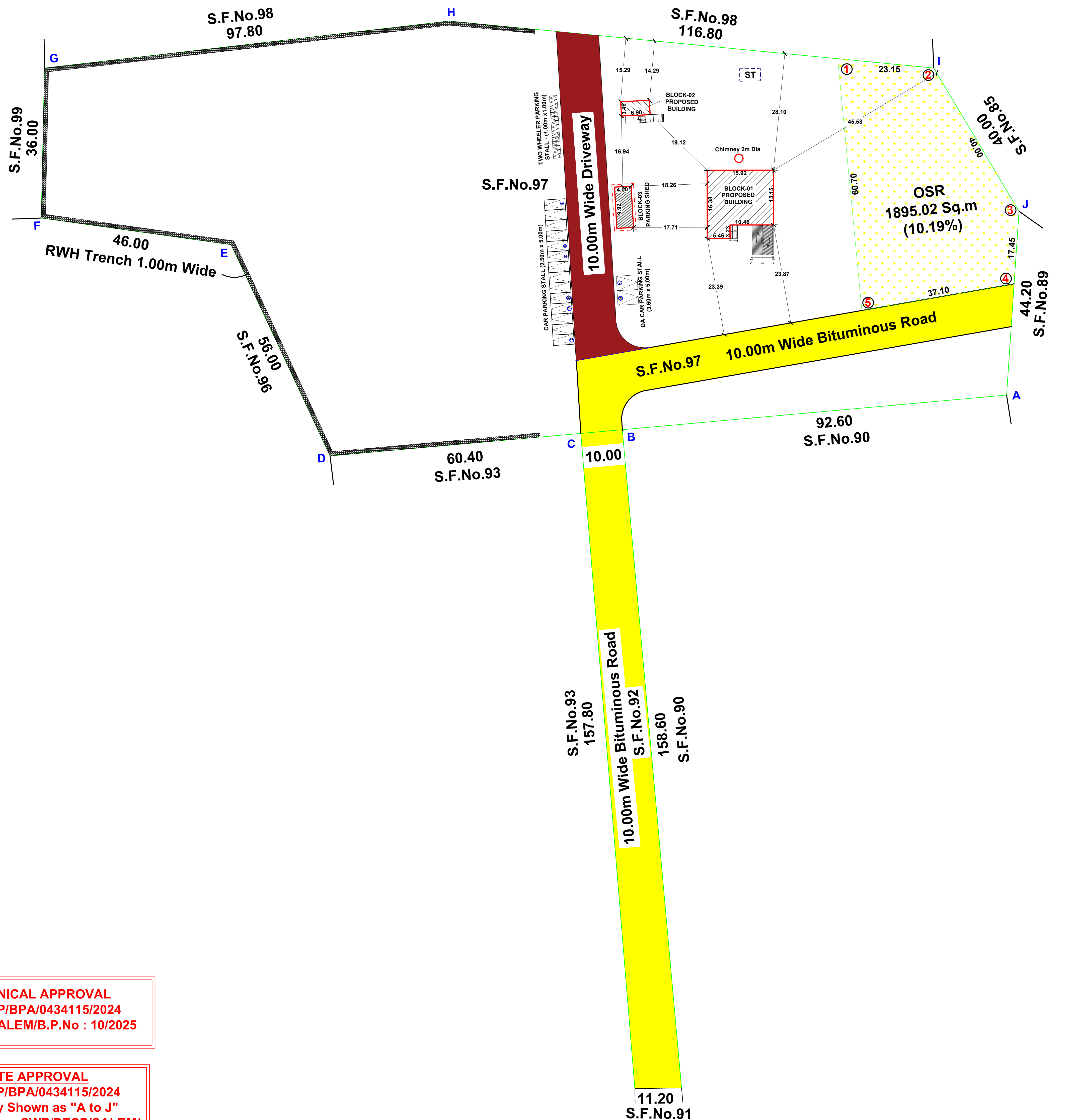
SITE PLAN SCALE - 1:400
