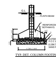
TYP. DET. COLUMN FOOTING
