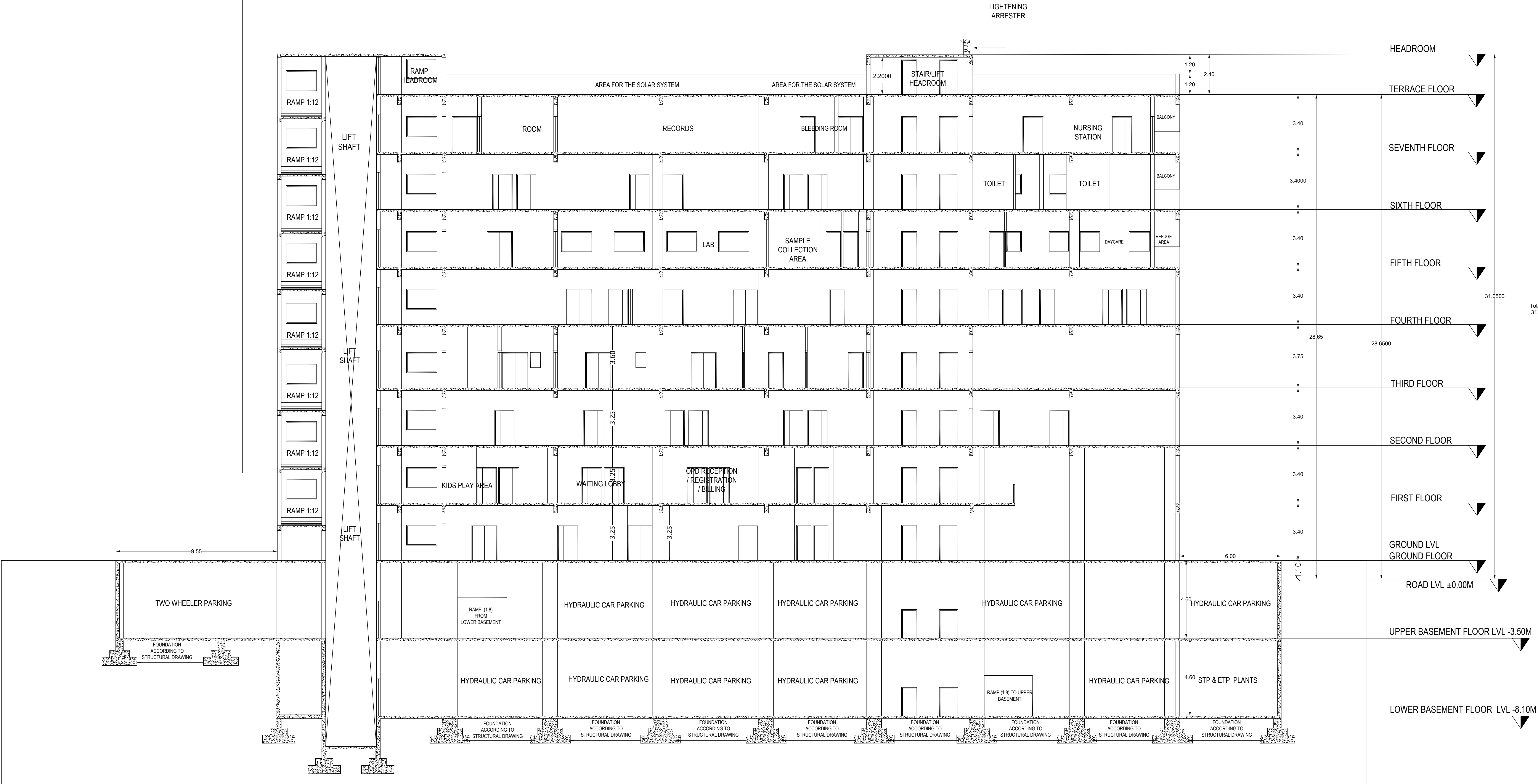
SECTION A-A'
