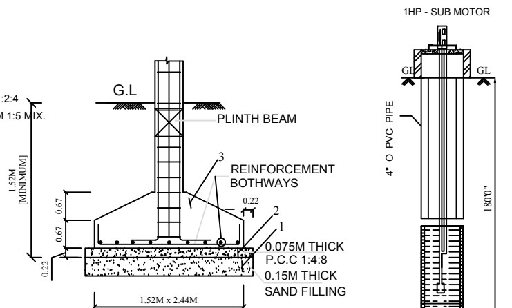
TYP. DET. COLUMN FOOTING
