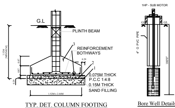
TYP. DET. COLUMN FOOTING
