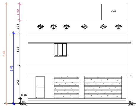
ELEVATION-A
