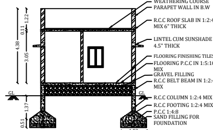
SECTION A-B
