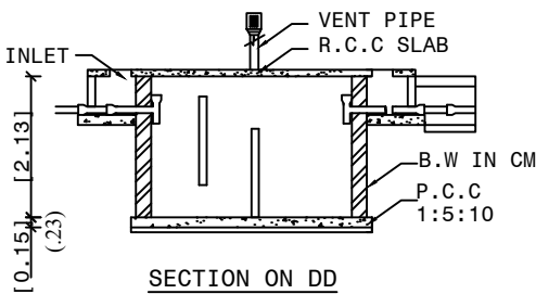
SECTION ON DD
