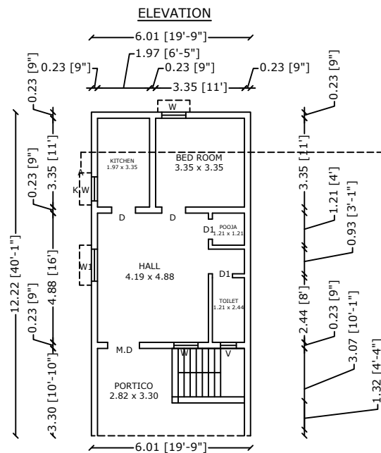
ELEVATION
