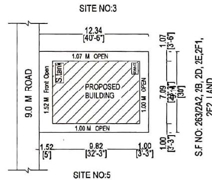
SITE PLAN (SCALE 1:200)
