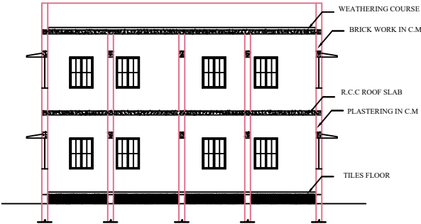
SECTION 'ab'
