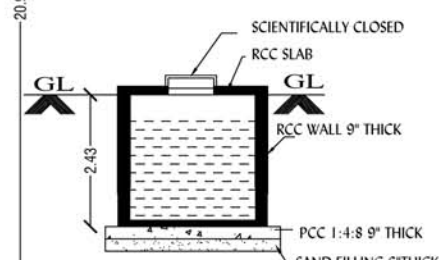
SEC -XX
