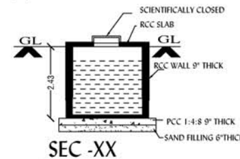
SEC -XX
