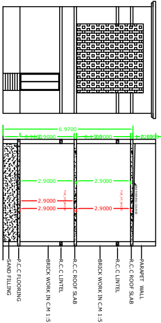
ELEVATION
