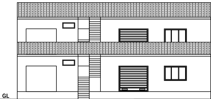
ELEVATION
