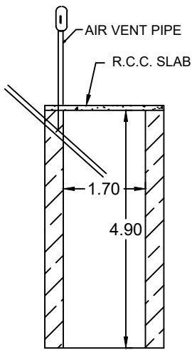
SOAK PIT
