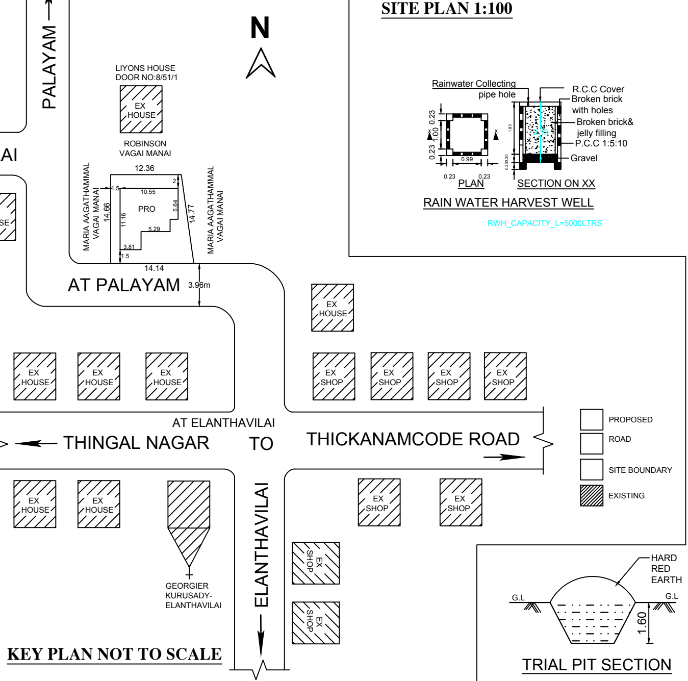
SITE PLAN 1:100
