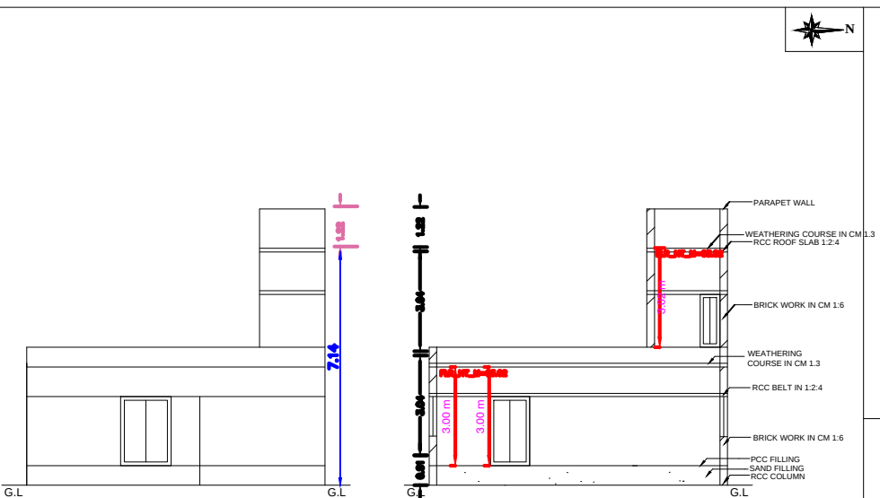
ELEVATION
