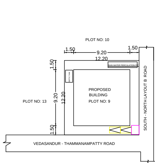
SITE PLAN : (SCALE 1:400)
