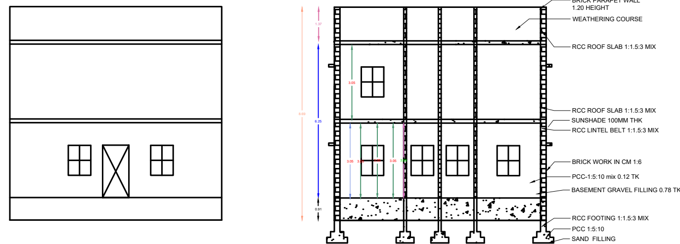
ELEVATION
