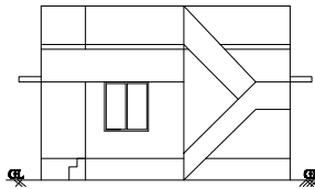
ELEVATION
