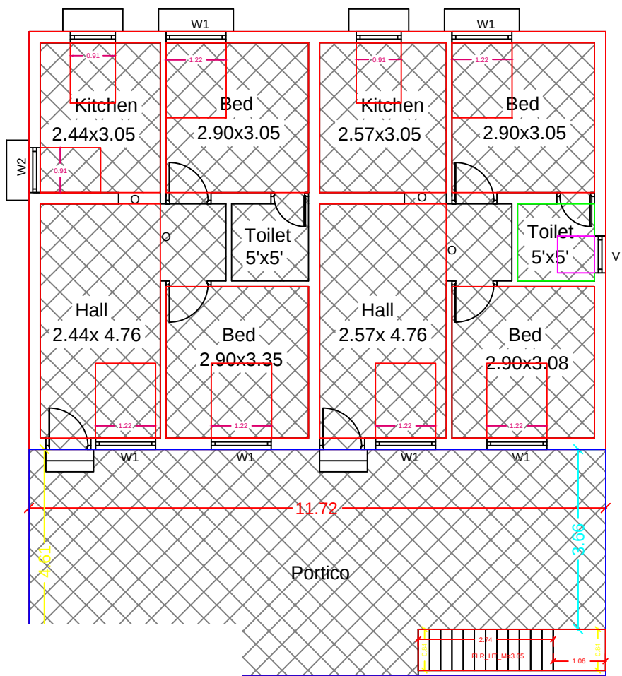
UND FLOOR PLAN
