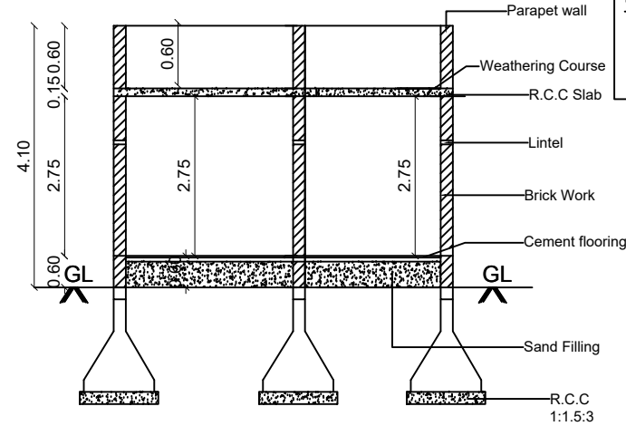
SECTION ON'AB'
