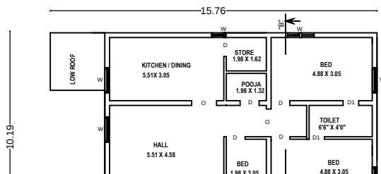
PRO. ALT. & ADD G.F PLAN
