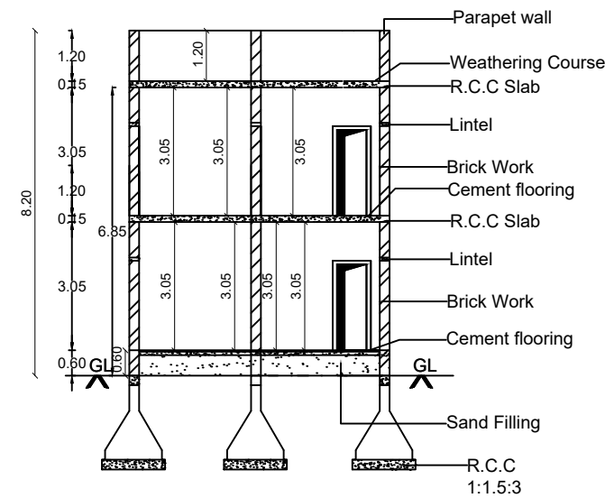
SECTION A-B
