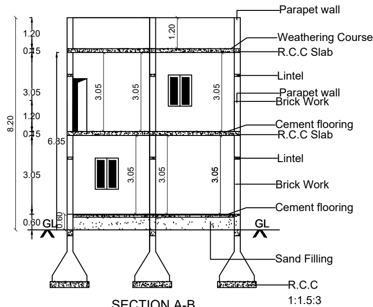
SECTION A-B
