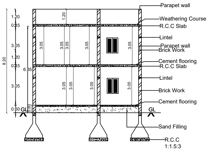
SECTION ON'AB'
