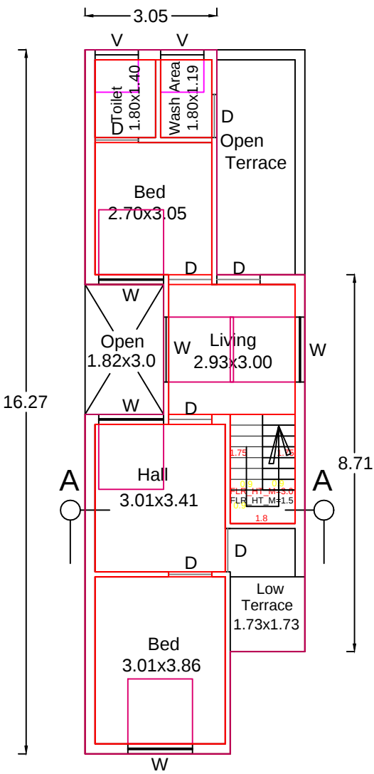
PLAN - F.F
