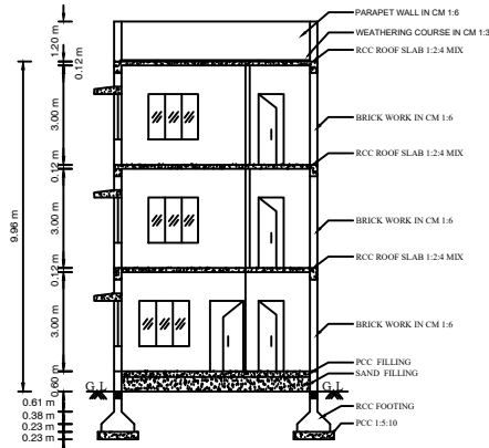
SECTION - AB
