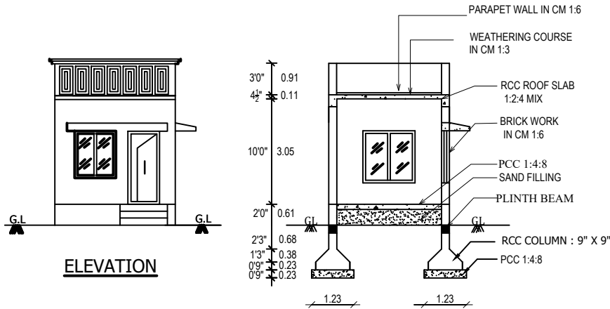
SECTION - AB
